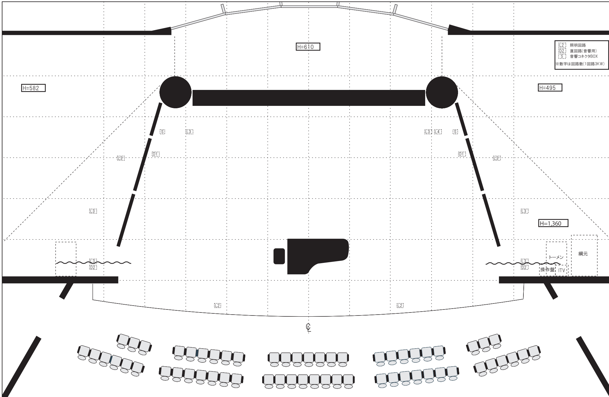
図面9 反響板(ピアノ有り)平面図
