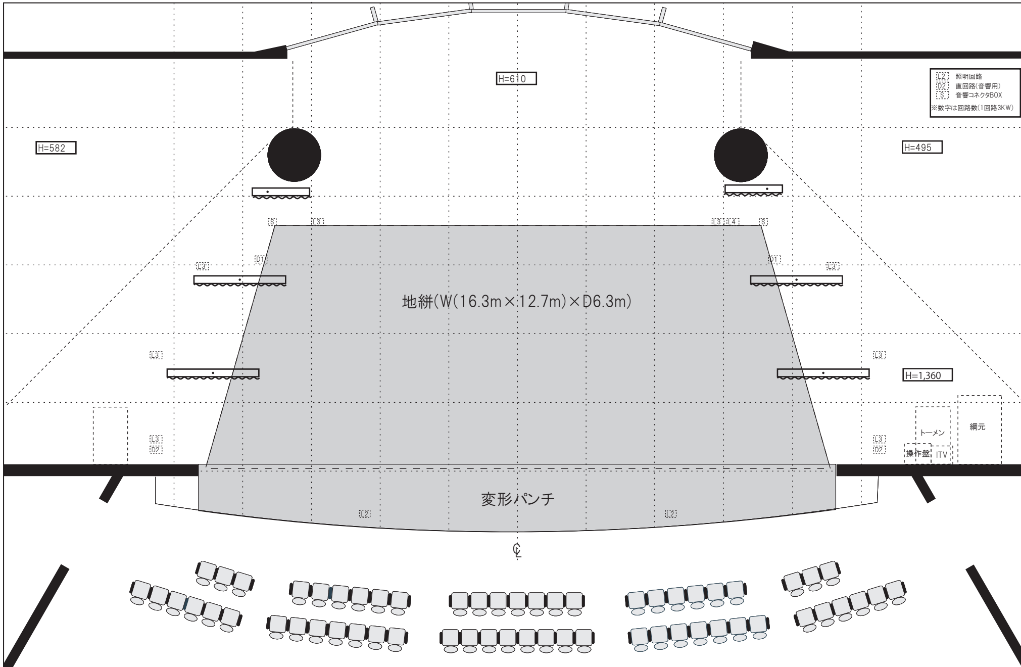
図面8 地絨敷込み図
