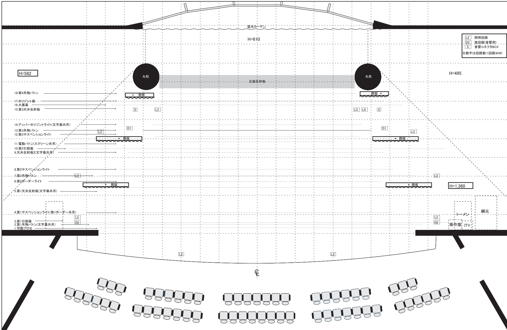
図面3 舞台平面図(1m単位)
