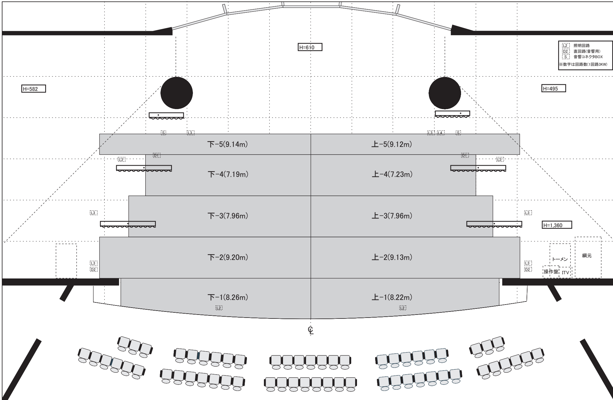
図面10 バレエ用シート敷込み図
