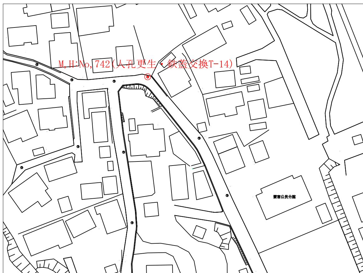
平面図 S=1:2,000
