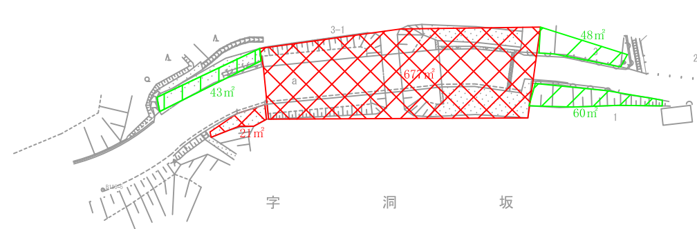
⑥飛ヶ崎トンネル
