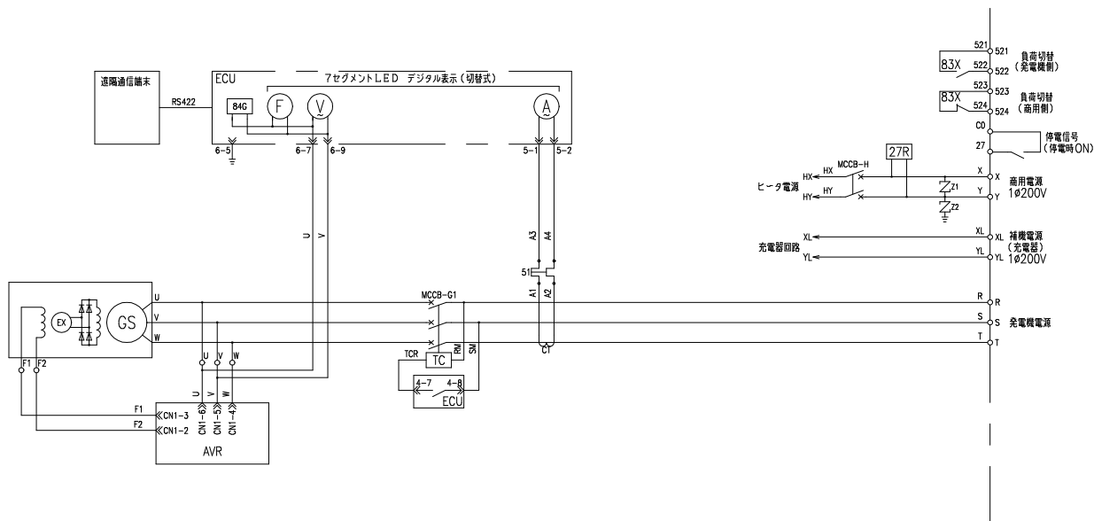
結線図
