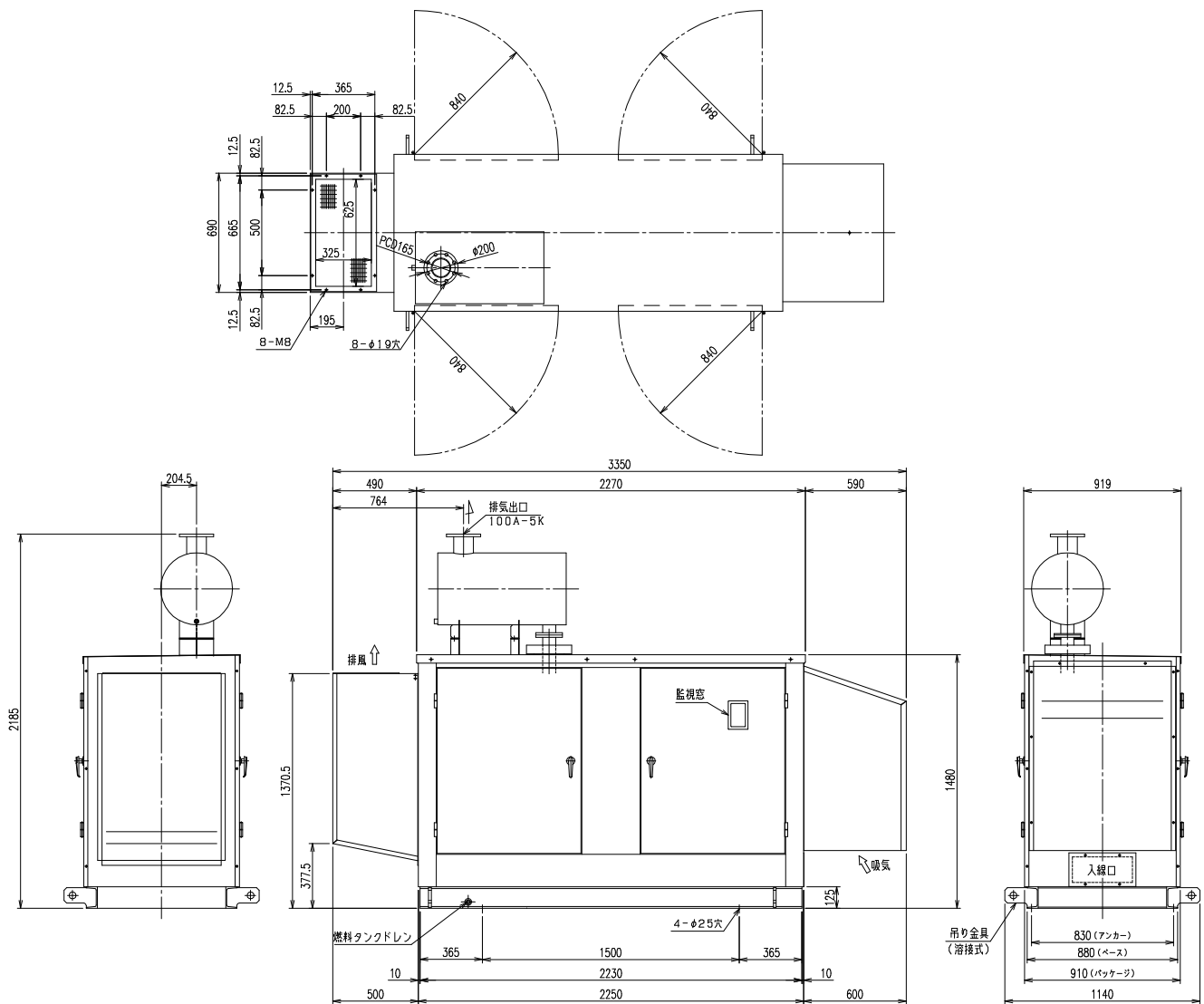
発電設備外形図 (S=1/40) (屋内仕様)
