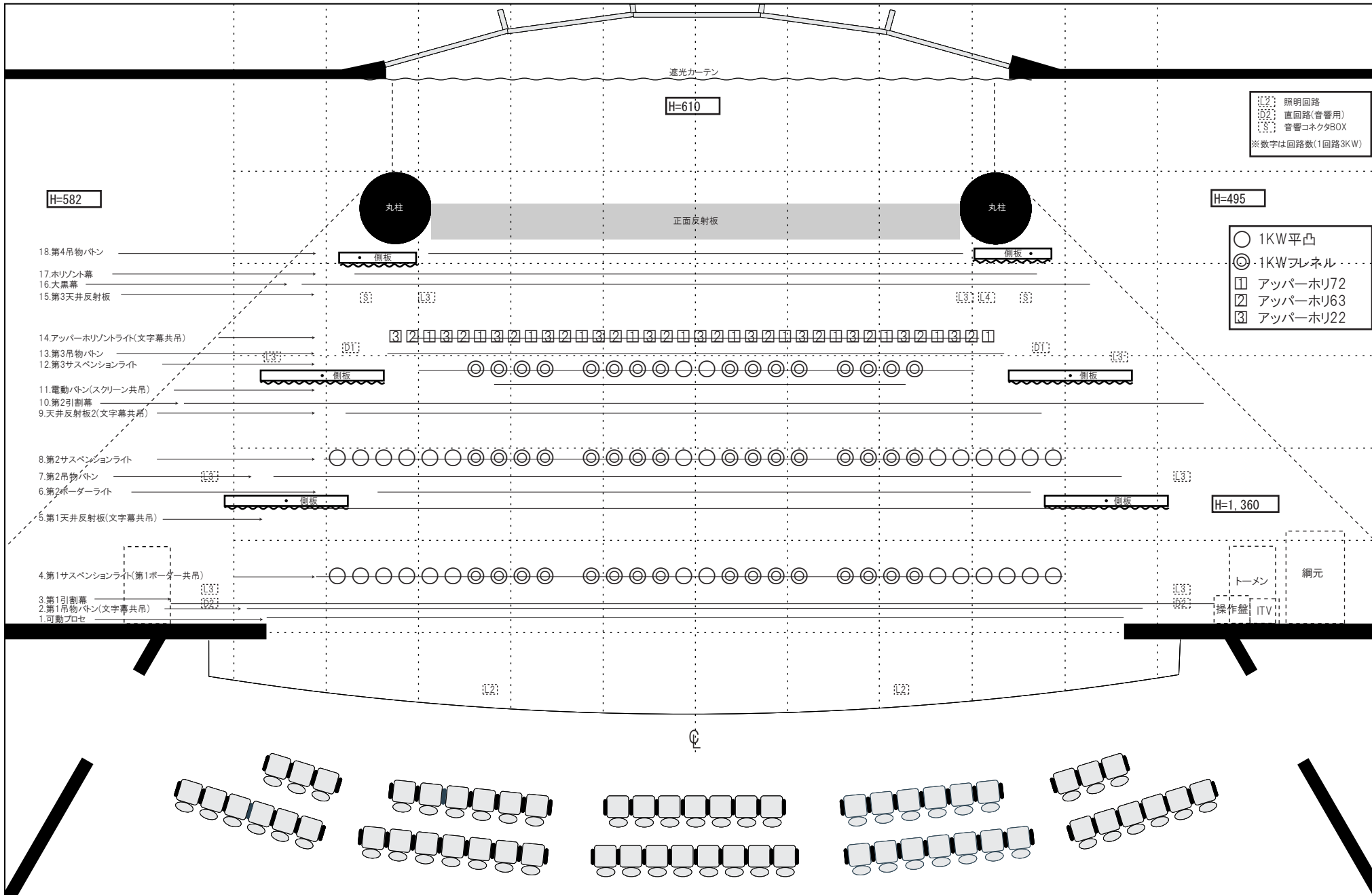
図面7 舞台照明標準吊込み図
