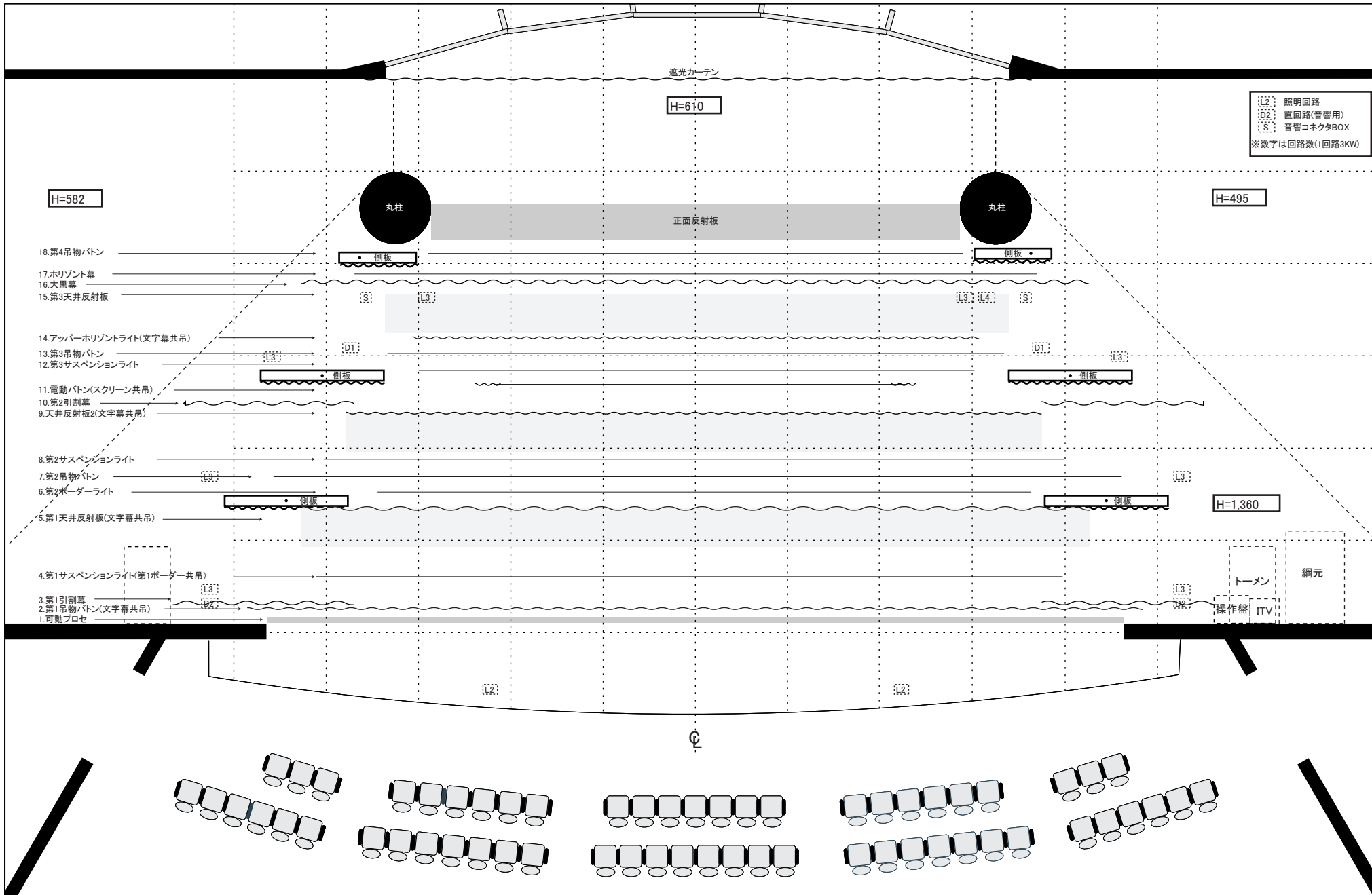
図面5 舞台吊物図
