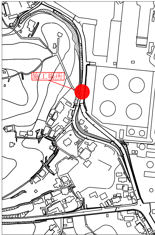
平面図(代ヶ崎) S=1:600
