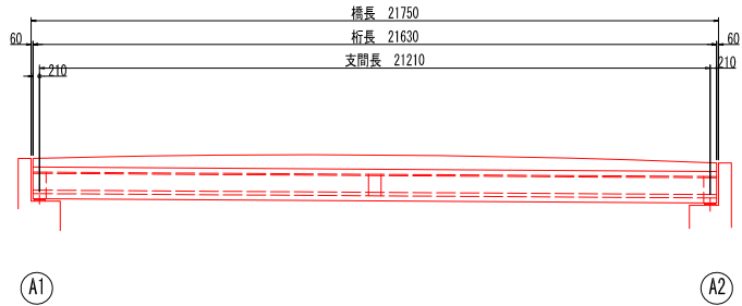
平面図
