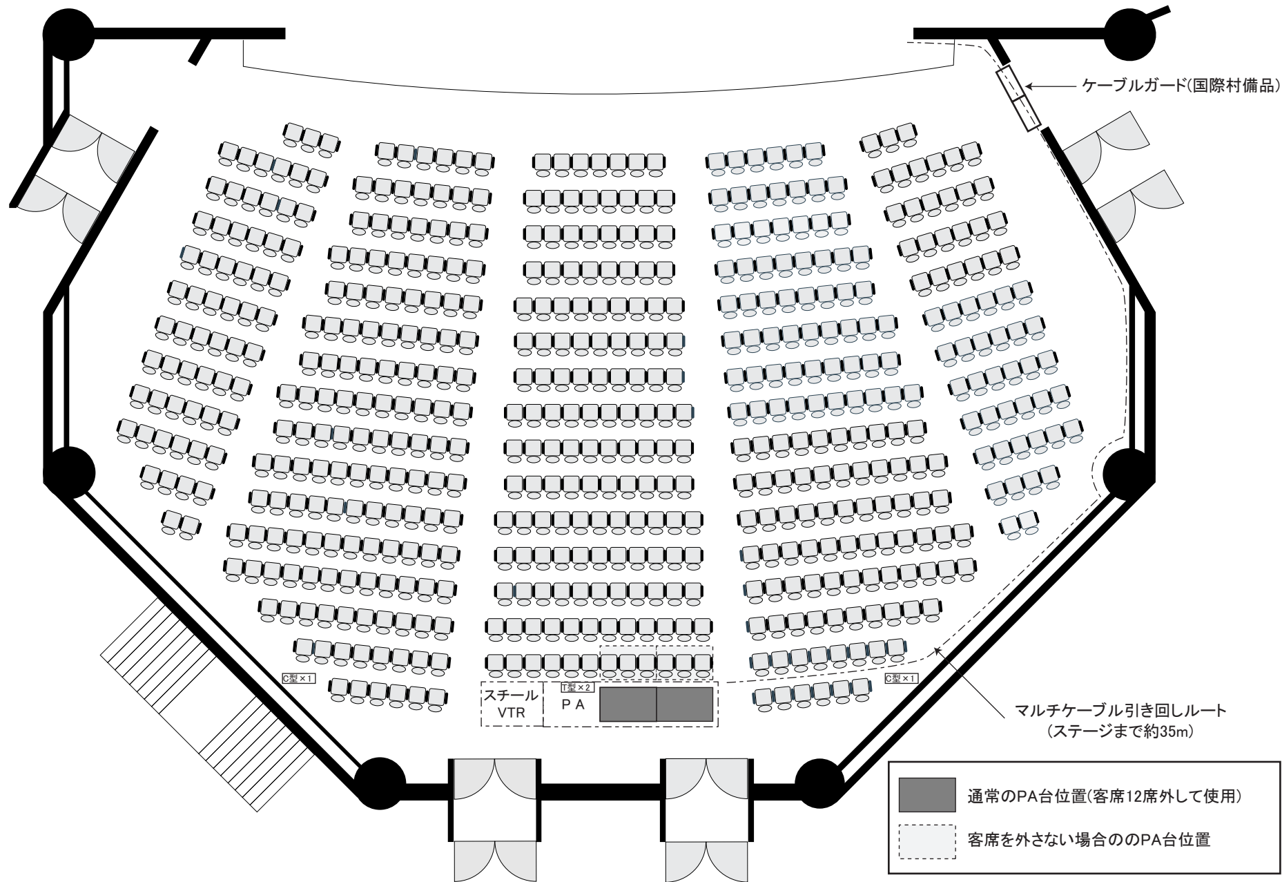
図面6 PA台位置図
